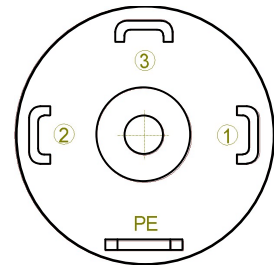
Versione ET- 521 Scatola di connessione
