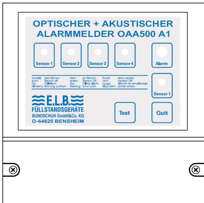
Dimensioni Alloggiamento: 137 mm x 186 mm (senza passacavo filettato) x 103 mm
